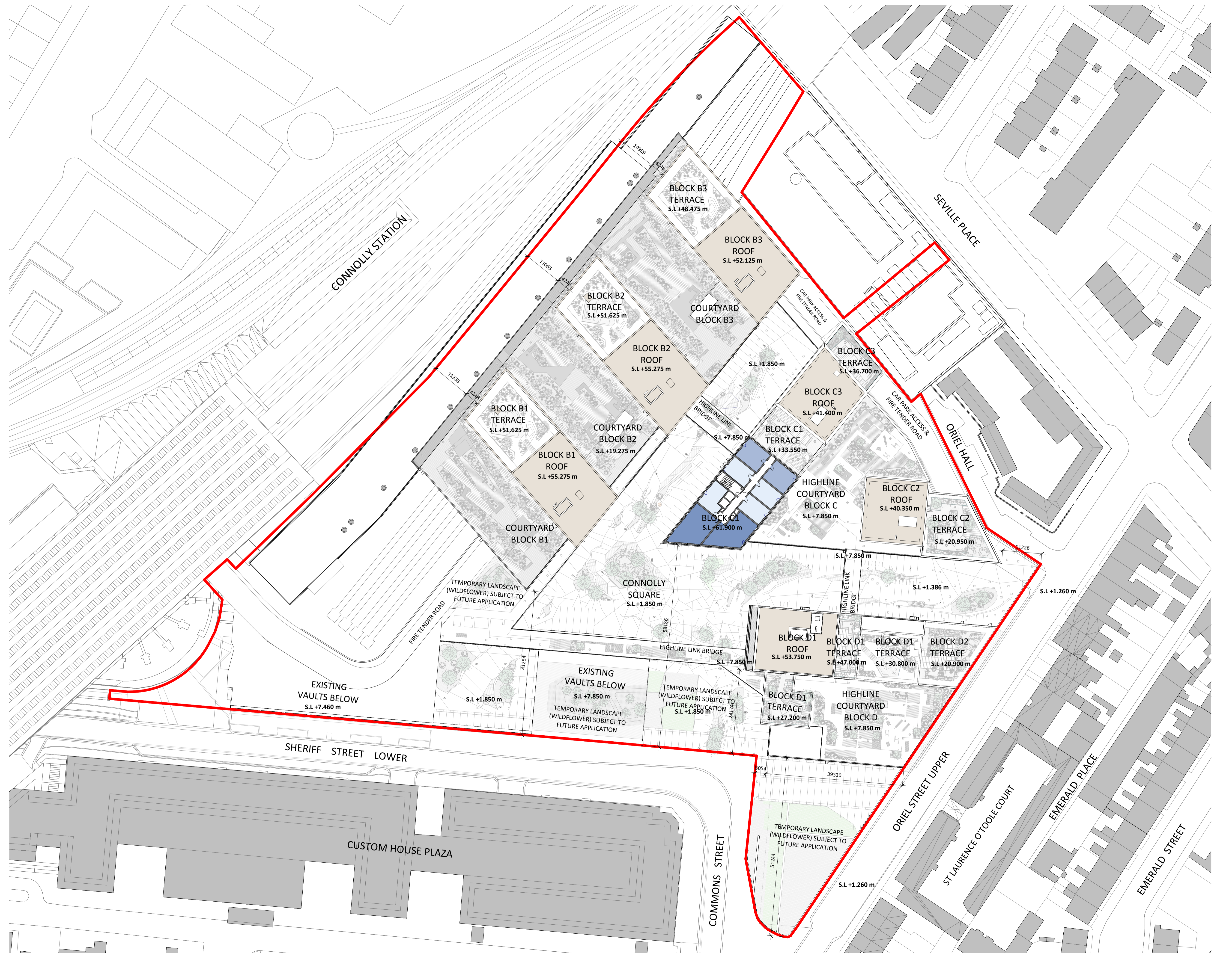
1 SITE LAYOUT PLAN - LEVEL 18 1 : 500
